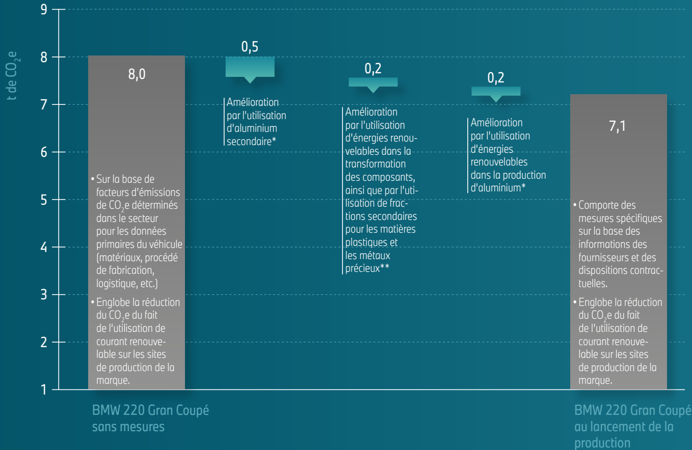
Fig. 5 : Influence des objectifs de développement sur le potentiel d'effet de serre de la phase de fabrication de la BMW 220 Gran Coupé
