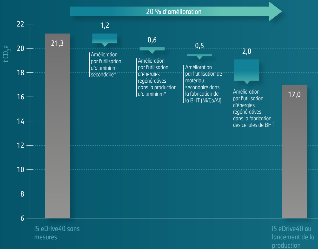
Fig. 5 : Influence des objectifs de développement sur le potentiel d'effet de serre de la phase de fabrication de la BMW i5
